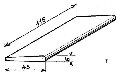
Couteau champ rond
