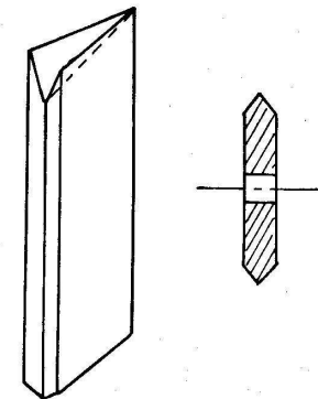
Outil pointu vertical et meule borazon pour dito
