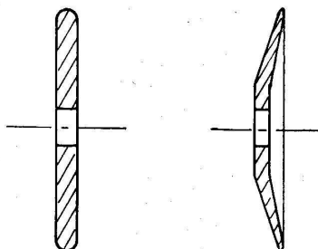
Meules demi-rondes Ø 175 x 30 x 8 Ø 200 x 30 x 14
